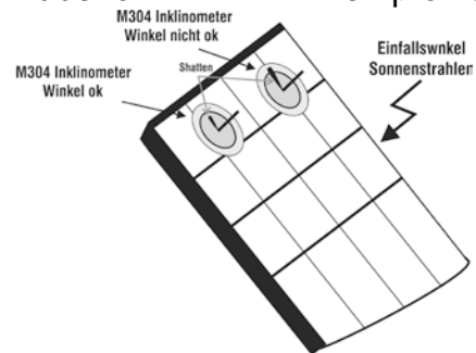
Abb. 7b: Positionierung des Inclinometers M304
