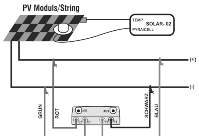
Abb.9: Anschluss des Messgerätes und SOLAR-02 an den String
