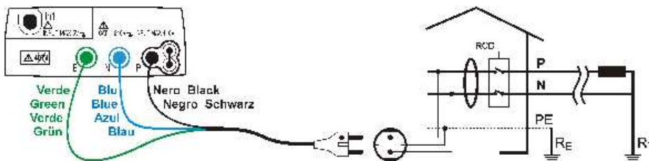
Abb. 4: Geräteanschluss mittels Schuko-Adapterkabel C2033x
