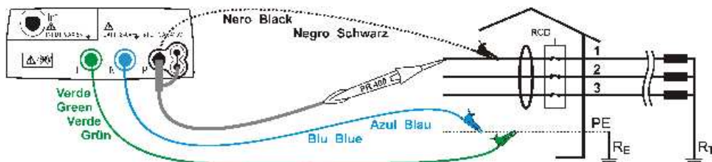
Abb. 23: Geräteanschluss zum 400V + PE (ohne N) dreiphasigen Messung des P-PE Schleifenwiderstandes mittels Einzelkabeln und Tastkopf
